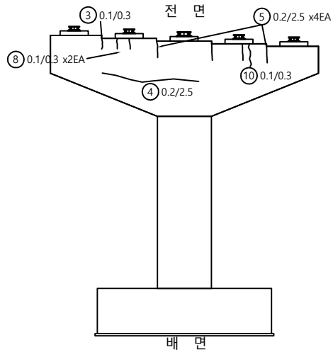
배면
