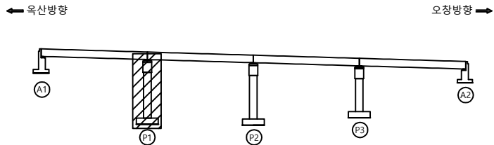
배면
